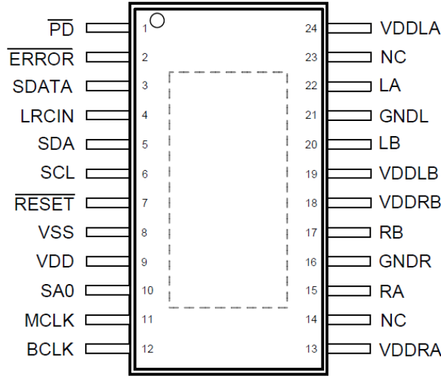
E-TSSOP-24L
